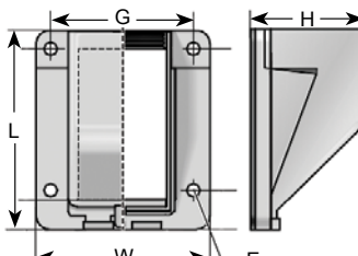
Flange Type 2: Conduit Size 29 - 48
